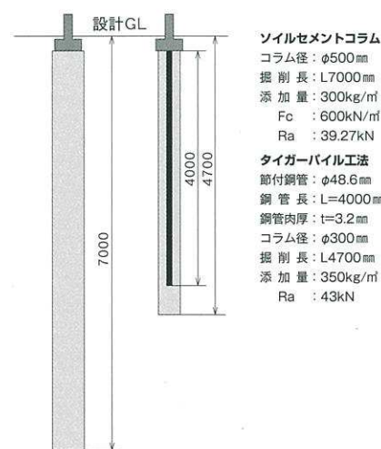
ソイルセメントコラム タイガーパイル
